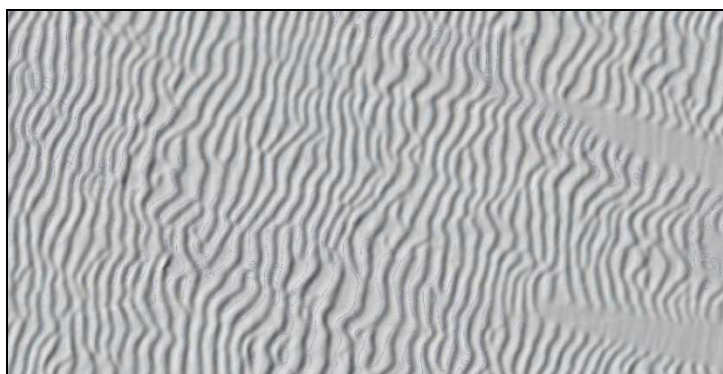
Рис. 1. Поле мегарифелей на площади КГКМ
